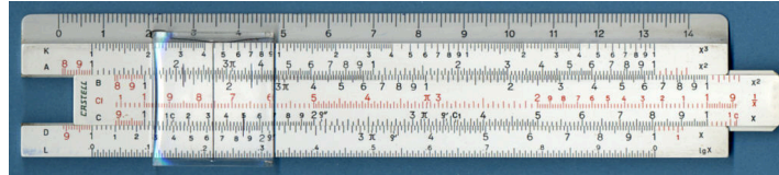
Slika 13.2 Drсно računalo. Osnovni skali sta D in drseči C. Računalo kaže produkt 1,24 \cdot 1,32 = 1,64 . Hkrati kaže kvocient 1,64/1,32 = 1,24 . Skala A je kvadrat skale D in kaže 1,64^2 = 2,7 oziroma \sqrt{2,7} = 1,64 . Podobno velja za skalo K, ki je kub skale D. Skala L pa je logaritem skale D in kaže \lg 1,64 = 0,215 . (Anon)
